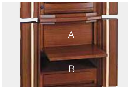
下台引出し1杯 供物棚スライド式 ※下台有効収納スペース (A) 高:16.5cm 幅:37cm 奥:27cm (B) 高:13cm 幅:42cm 奥:37cm 供物棚の奥に隠しBOX付
