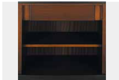
下台引出し1杯/棚1枚 ※下台有効収納スペース(棚取り外し時) 高:37.5cm 幅:42cm 奥:39.5cm
